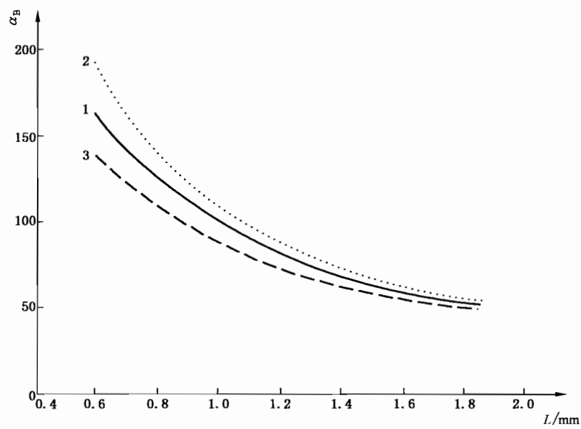
图 A.1 表明了抗压痕性作为压痕长度(取最小分度 \Delta L 为 0.1 mm)的函数计算误差。
